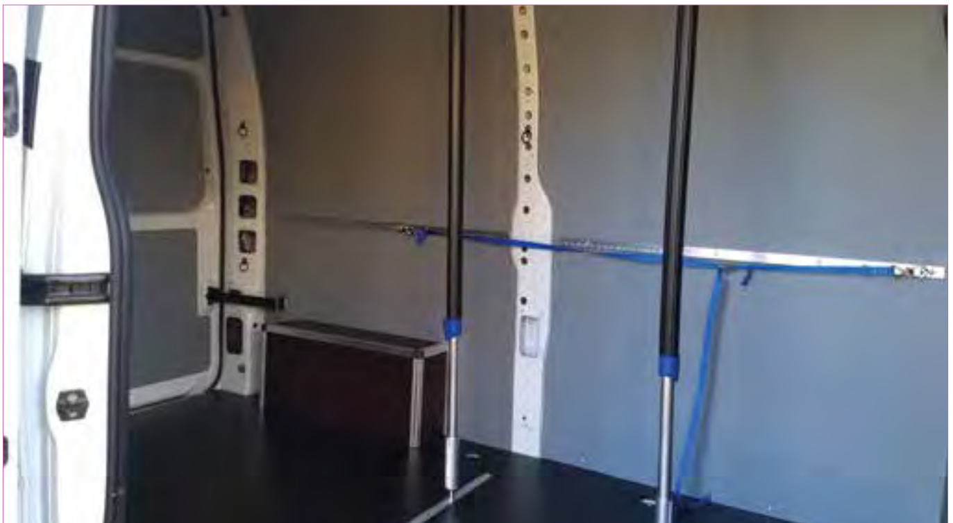
Vloerplaat en wanden met vastzetrails
